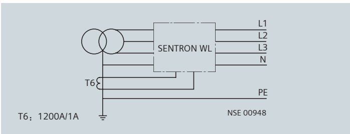
4 极断路器，电流互感器位于星形接地点
