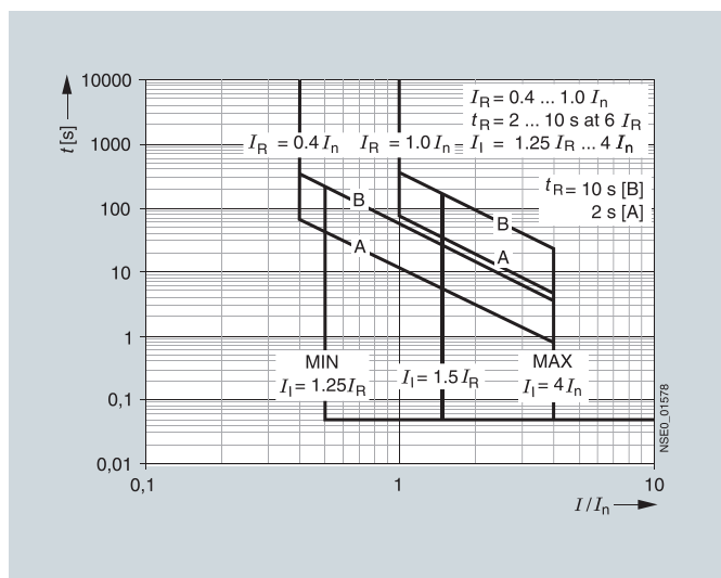
DIGmat S100 控制器特性曲线
