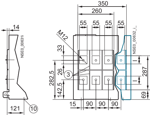
法兰连接
