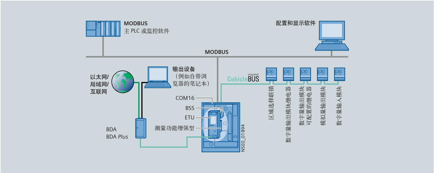
与 MODBUS 通讯
