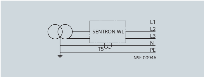
3 极断路器，中性线上的电流互感器
