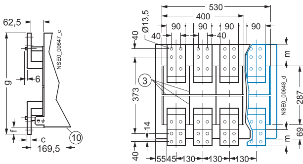
法兰连接
