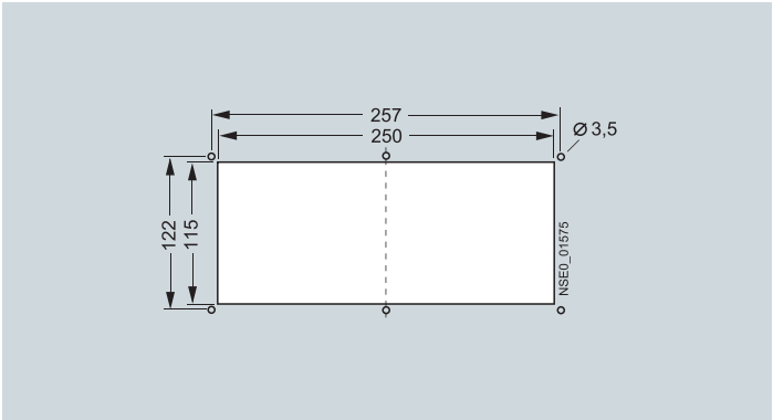
DIGmat S100 控制器器钻孔图
