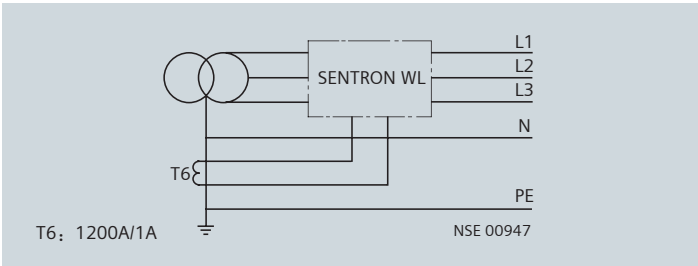
3 极断路器，电流互感器位于星形接地点
