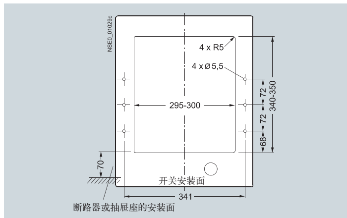
带 IP55 保护盖的操作面板柜门开孔
