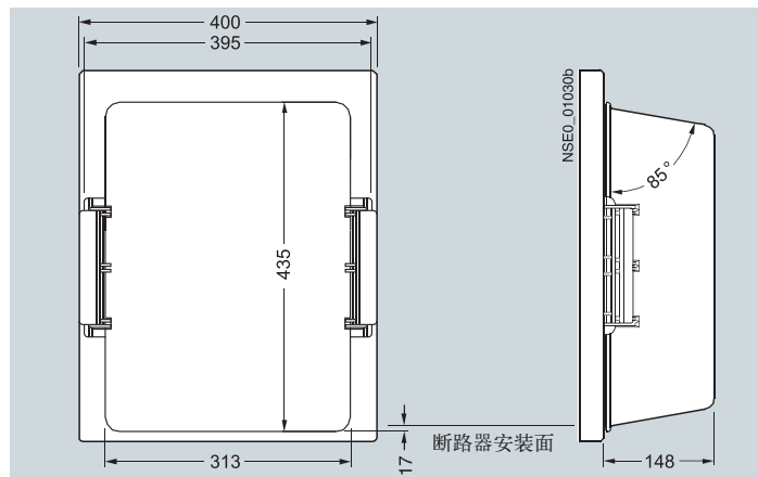
防护罩, IP55
