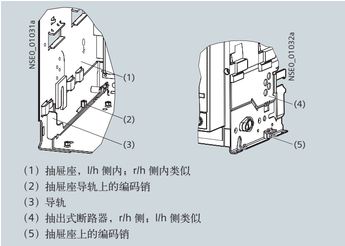
断路器与抽屉座之间的额定电流编码
